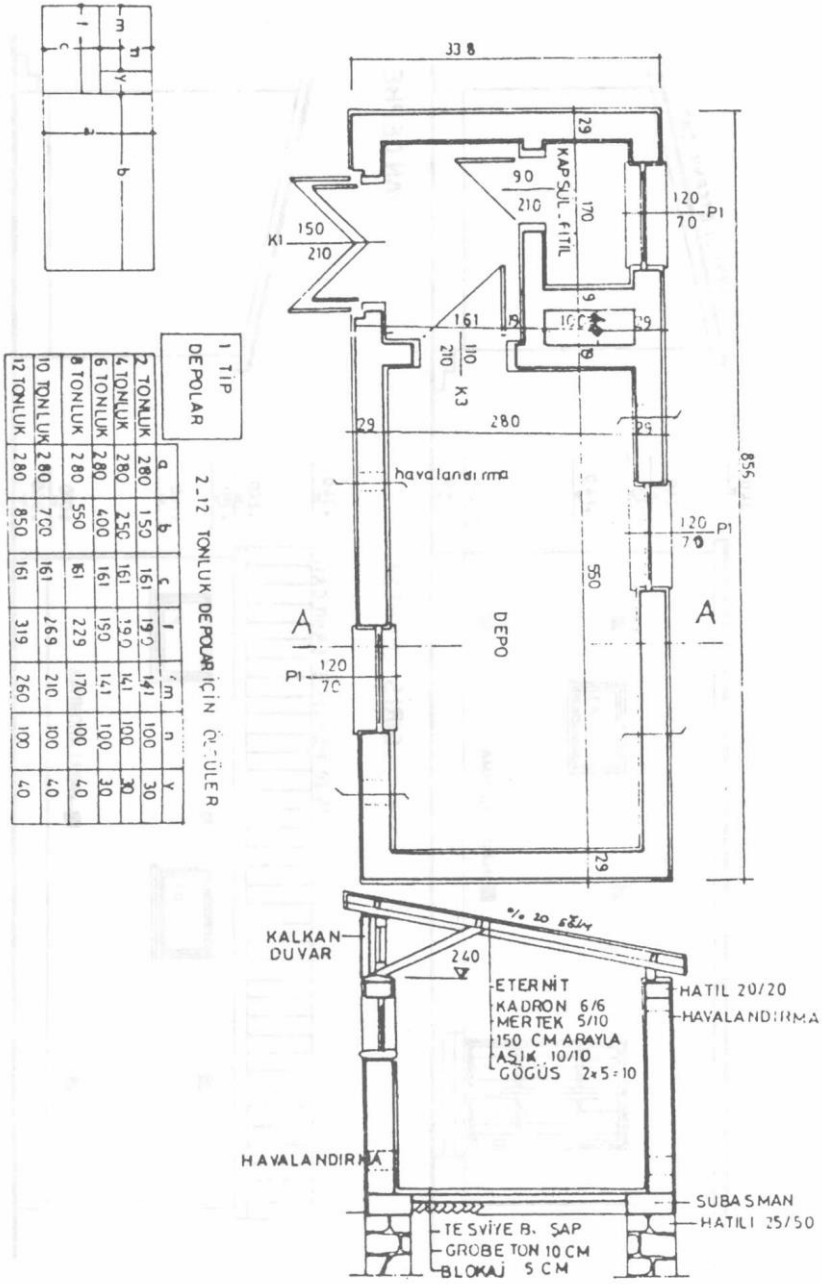
A-A Kesiti
